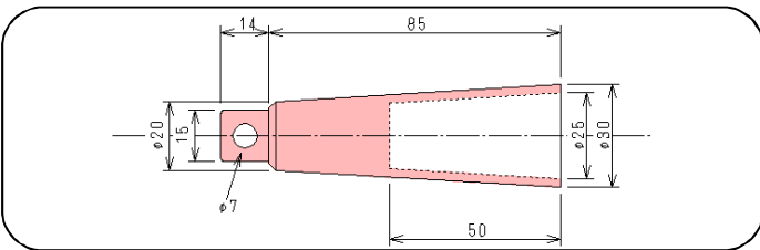
1)環式200g真鍮製テーパー分銅(下部空洞有り)
