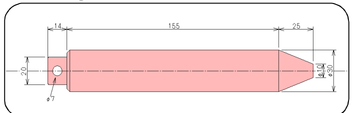
4)環式1kg真鍮製分銅
