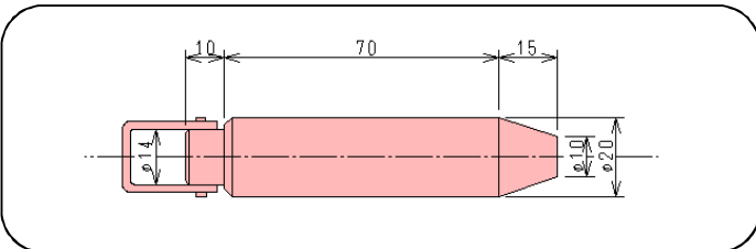
3)直結式220g真鍮製分銅
