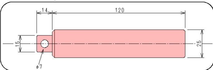
3)環式500g真鍮製軽油分銅
