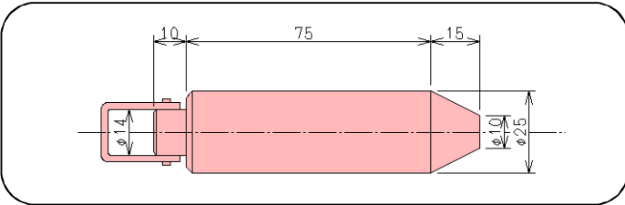
1)直結式350g真鍮製分銅(標準分銅)
