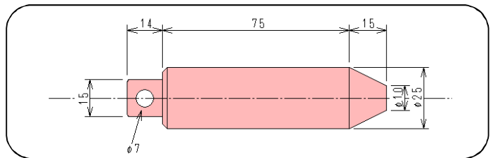
2)環式350g真鍮製分銅
