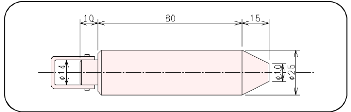
2)直結式350gステンレス製分銅
