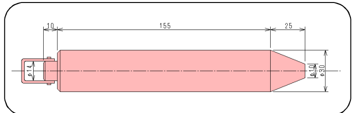
4)直結式1kg真鍮製分銅
